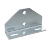
SSG-9G IFBL90D2AS165 Уголок L-образный, регулируемый, с 2 отверстиями
